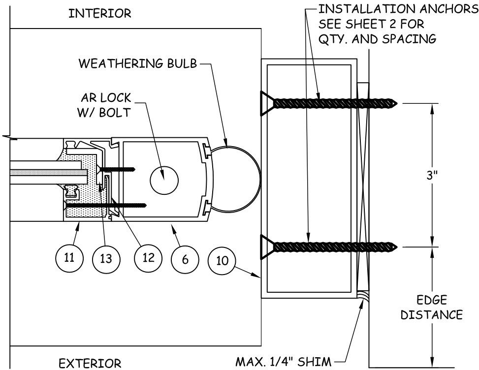
E 5 HORIZONTAL SECTION JAMB
